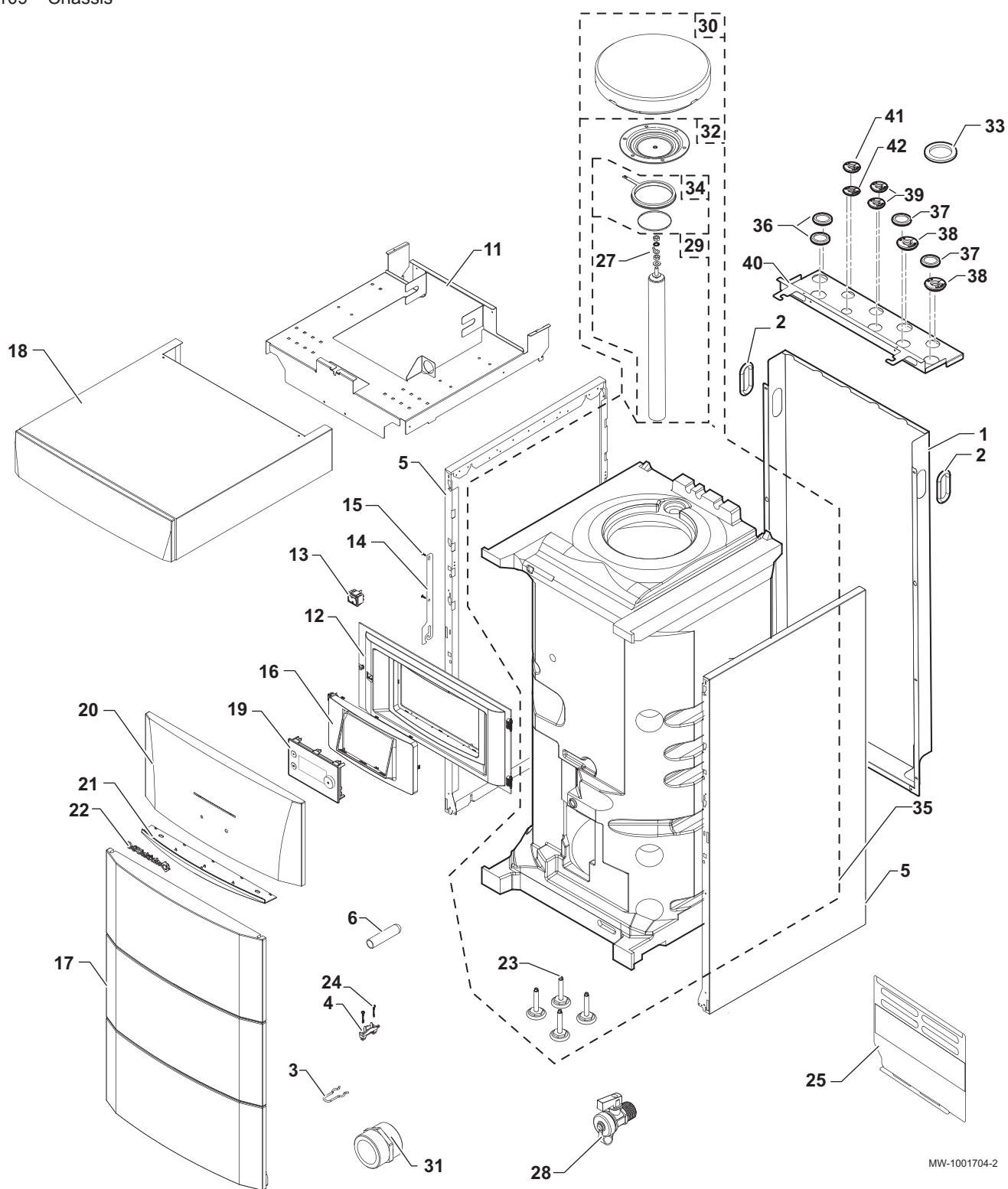
Fig.109 Châssis
