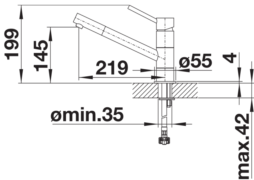
Vue latérale
