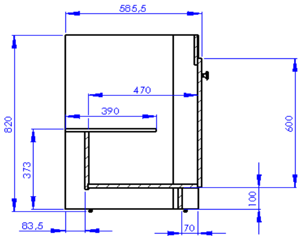
COUPE A-A
