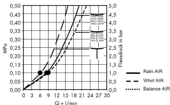
Le diagramme de débit : (avec filtre)
