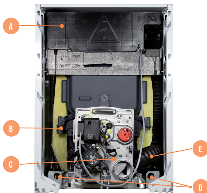
VUE AVANT MODÈLE CHAUFFAGE SEUL
