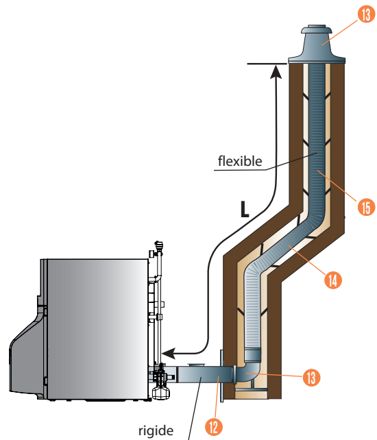
NOLEA EVO HTE 24-32 L Maxi = 7,7 m avec 1 coude 90° et 2 coudes 45°
