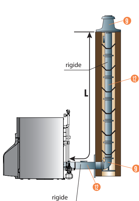
NOLEA EVO HTE 24-32 L Maxi = 13,1 m avec 1 coude 90°
