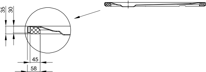
Présentation avec Support Minimum prémonté (T1).
