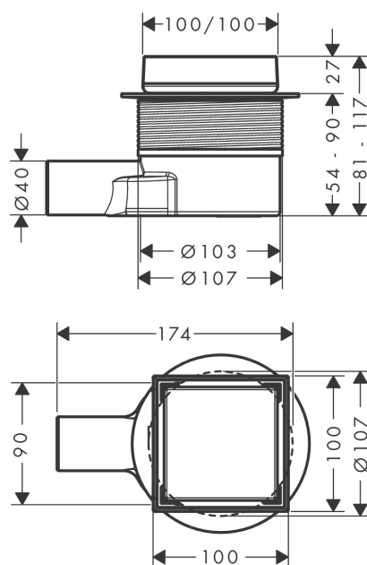
Plan géométral
