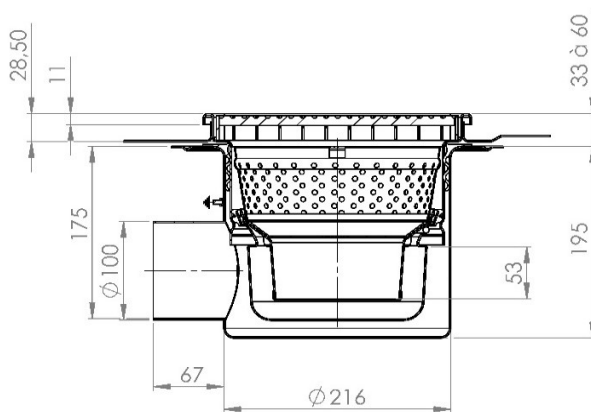
COUPE A-A
