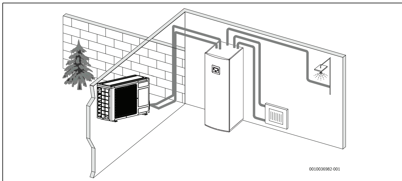
Fig. 2 La pompe à chaleur pour l'unité extérieure, l'unité intérieure AWS M avec un ballon d'eau chaude sanitaire intégré et le chauffage d'appoint électrique.
