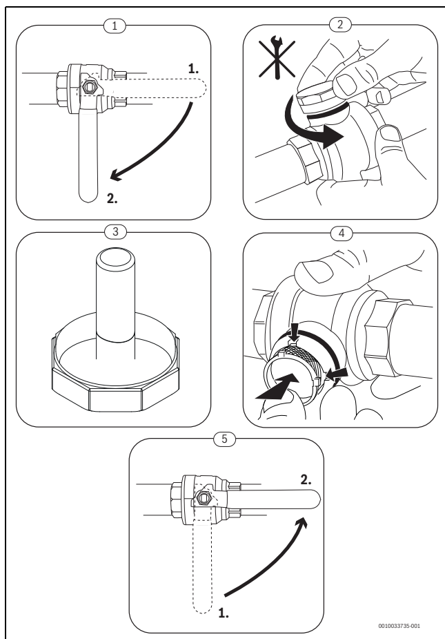
Fig. 5 Nettoyage du filtre
