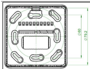
Dimension les plaques de base ClimaCon
