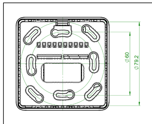
Dimension les plaques de base ClimaCon
