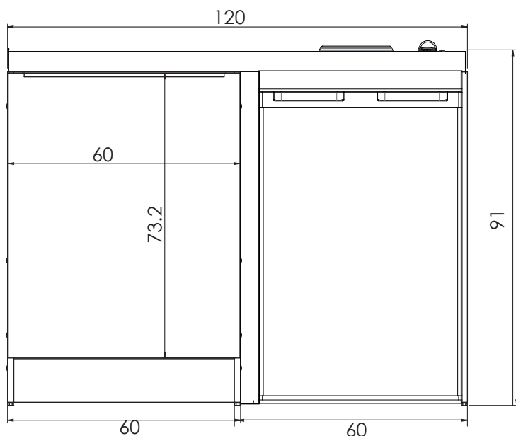
Vue face
