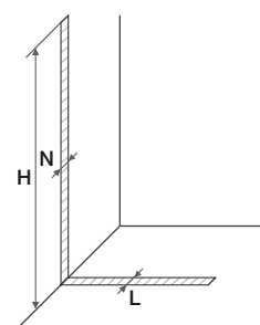
Réglage du faux-aplomb du mur
