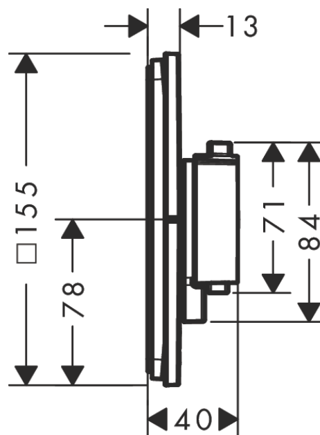
Plan géométral
