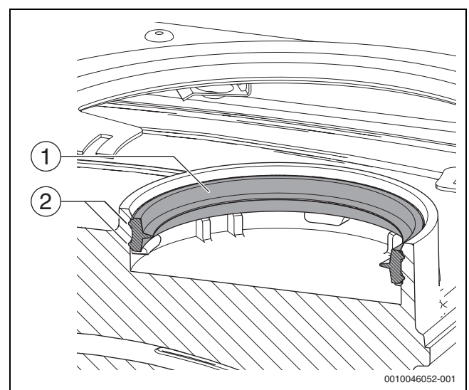
Fig. 137 Installer le joint à lèvres.
