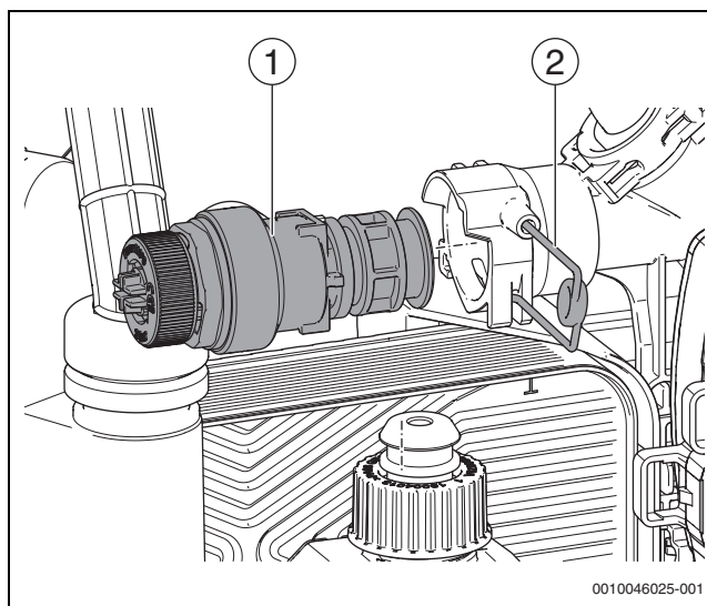
Fig. 146 Démontez la vanne de sécurité
