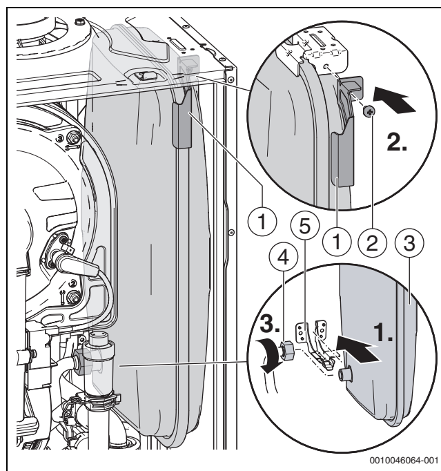
Fig. 139 Monter un nouveau vase d'expansion
