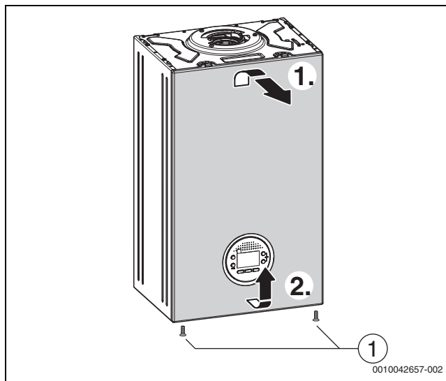
Fig. 21 Retirer l'habillage avant
