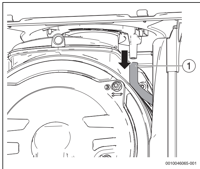
Fig. 60 Démonter le tuyau d'écoulement de l'eau
