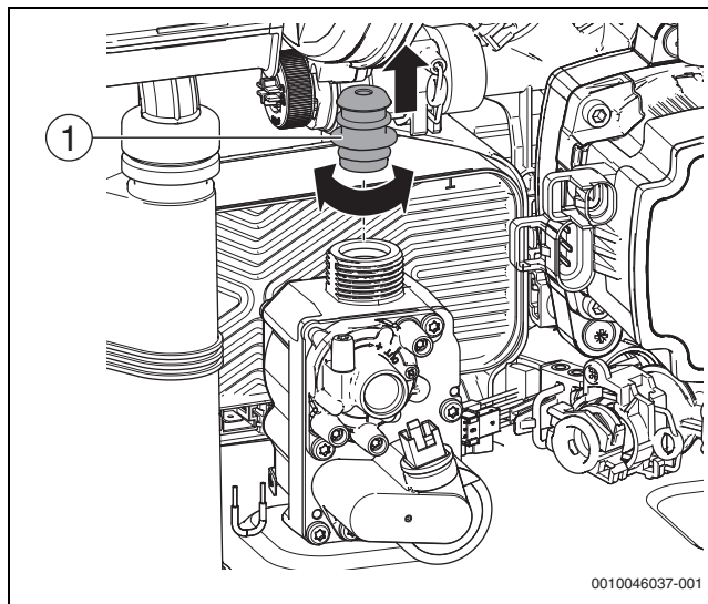
Fig. 123 Démontez le pré-étranglement
