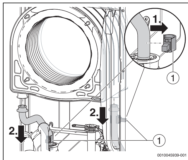
Fig. 104 Démonter les NTC et les tubes
