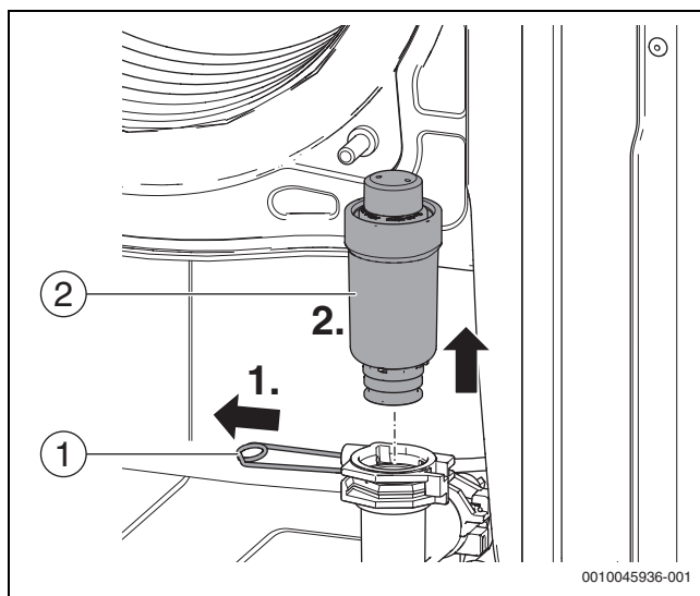
Fig. 101 Démonter le purgeur automatique
