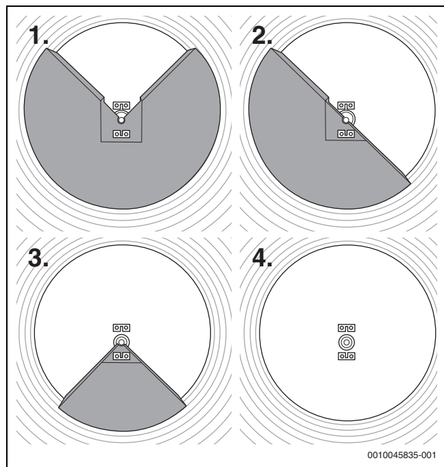
Fig. 74 Étapes de démontage de l'isolation
