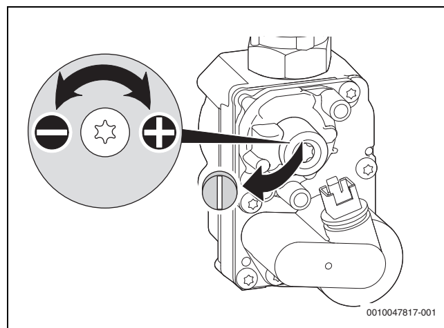
Fig. 40 Retrait du scellé de la vis de réglage
