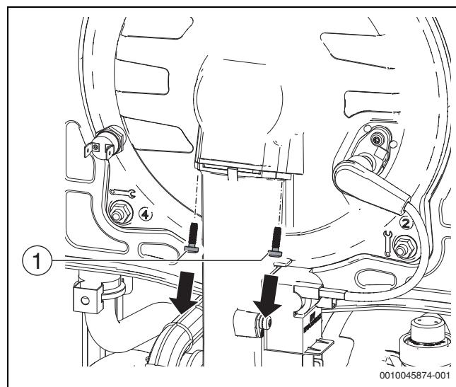
Fig. 80 Démontage des vis
