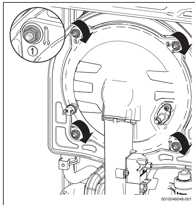
Fig. 129 Fixer le module de la porte foyer sur l'échangeur thermique
