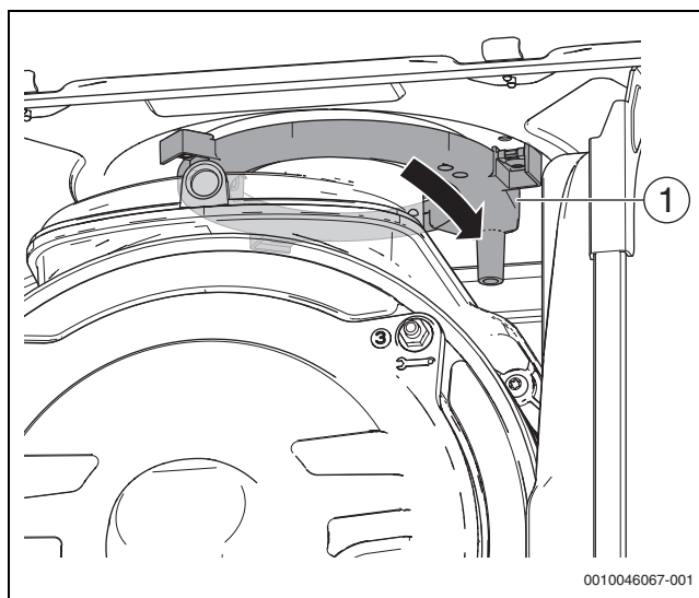
Fig. 62 Démonter la protection contre la pluie
