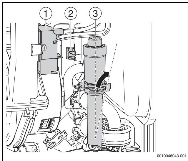
Fig. 132 Démonter les NTC sur le tuyau de retour
