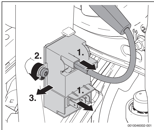
Fig. 109 Démonter le transformateur d'allumage
