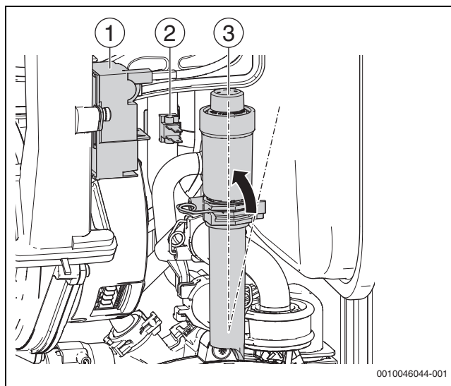
Fig. 133 Monter les nouveaux NTC sur le tuyau de retour
