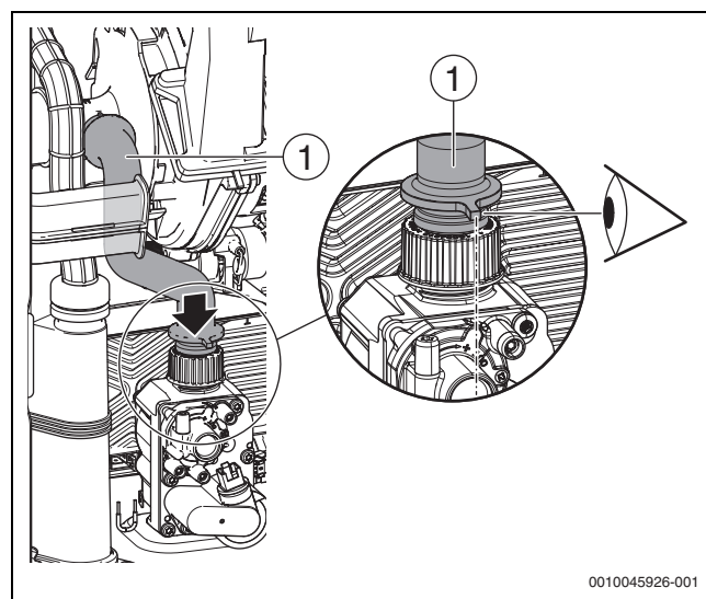
Fig. 97 Montage du tuyau de gaz
