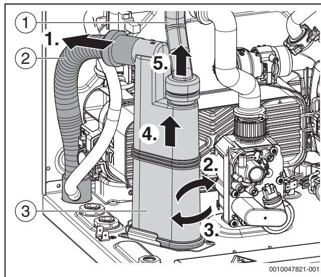
Fig. 55 Démontage le siphon des condensats
