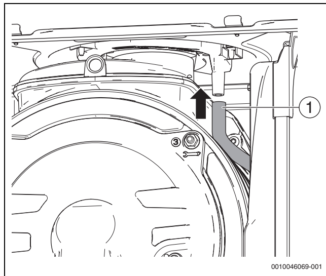
Fig. 65 Installer le tuyau d'écoulement de l'eau
