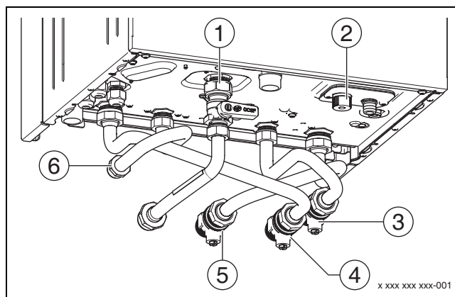
Fig. 24 Raccordement côté gaz et eau xDOS GA 6
