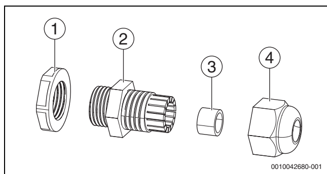
Fig. 30 Pièces du presse-étoupe
