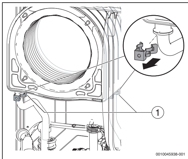
Fig. 103 Démonter les colliers
