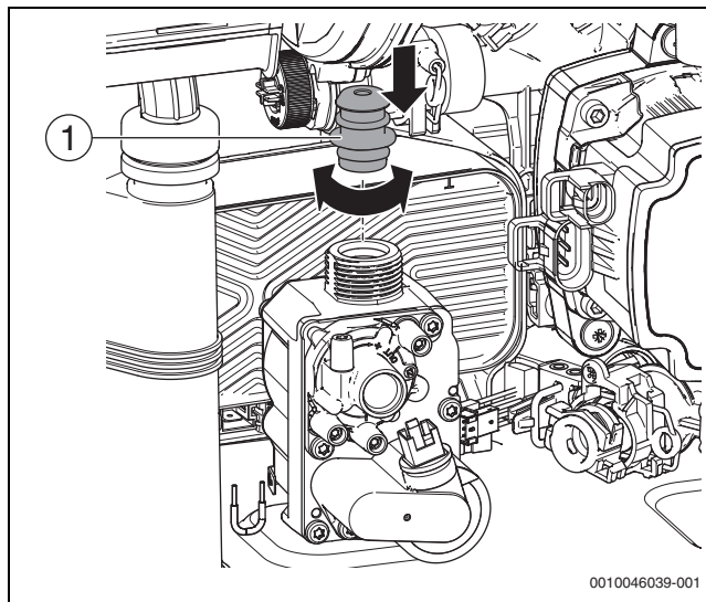
Fig. 125 Mettre en place le nouveau pré-étranglement et l'écrou de gaz
