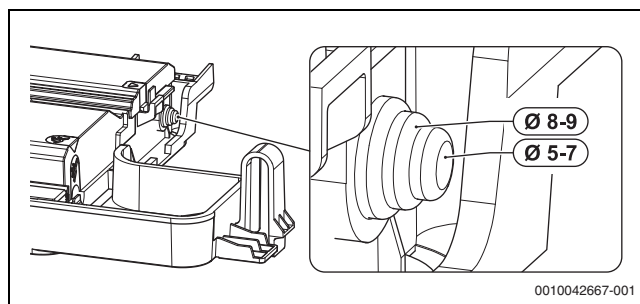
Fig. 33 Passe-câbles
