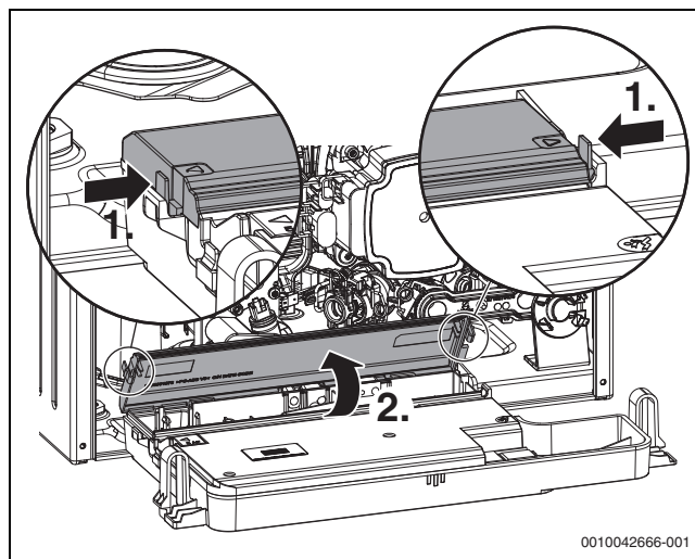
Fig. 32 Ouverture du couvercle de service
