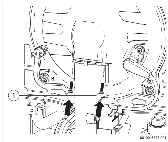
Fig. 88 Montage du tube d'air pour gaz sur la porte foyer
