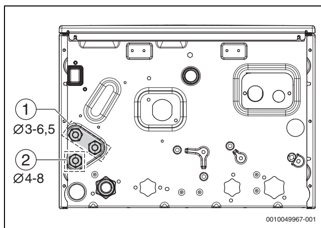
Fig. 29 Diamètre de câble
