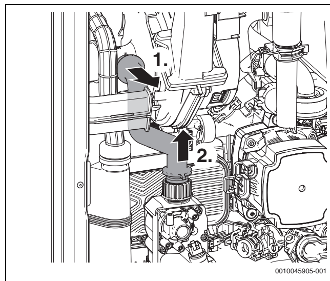
Fig. 89 Démontage du tuyau de gaz
