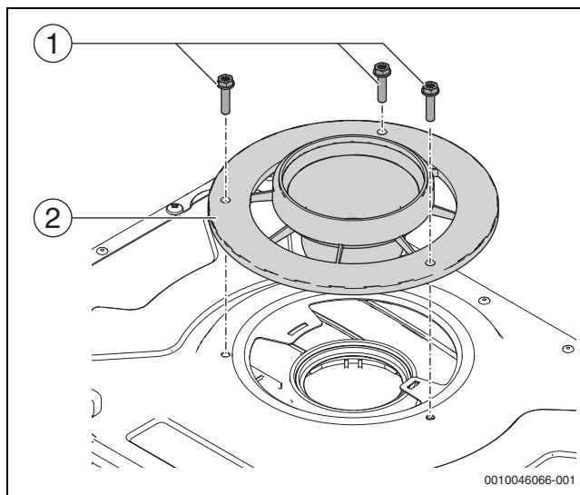
Fig. 61 Démonter le set du conduit de fumées et l'adaptateur du conduit de fumées
