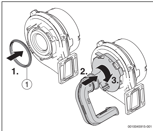
Fig. 92 Montage du ventilateur
