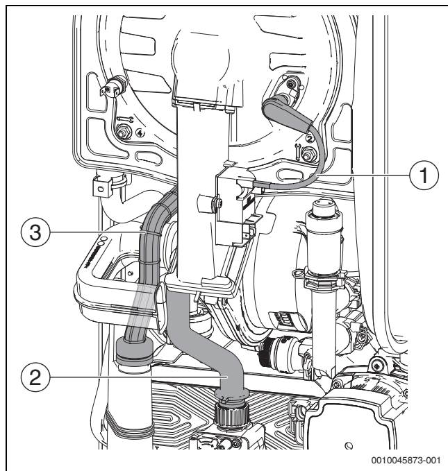
Fig. 79 Porte foyer
