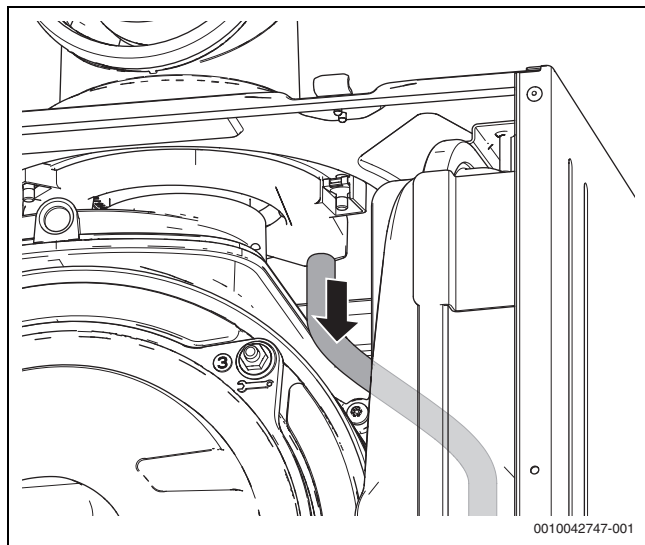
Fig. 148 Démonter le déflecteur de pluie
