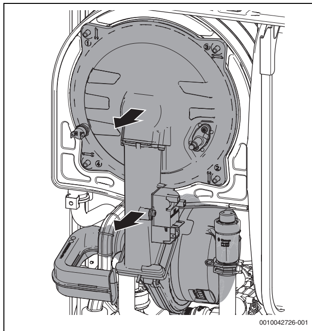
Fig. 100 Démonter le module de la porte foyer
