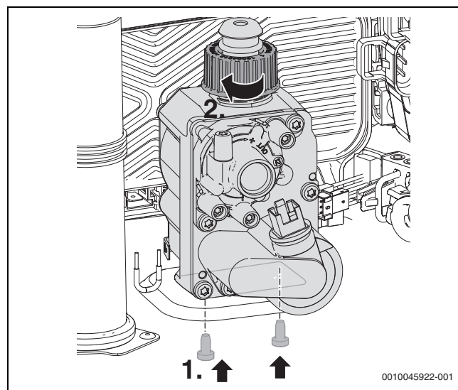
Fig. 96 Montage de la vis et de l'écrou
