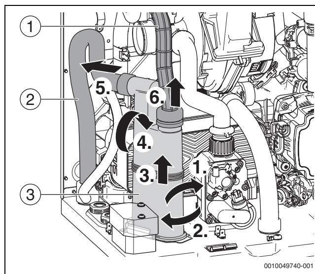
Fig. 56 Démontage le siphon des condensats
