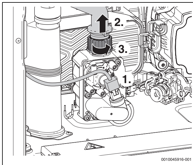
Fig. 93 Démontage du tuyau de gaz, du connecteur et de l'écrou
