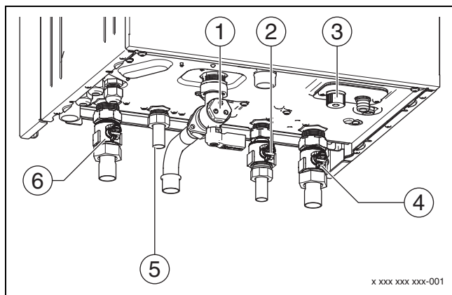
Fig. 23 Raccordement côté gaz et eau xDOS GA 5/xDOS GA 15
