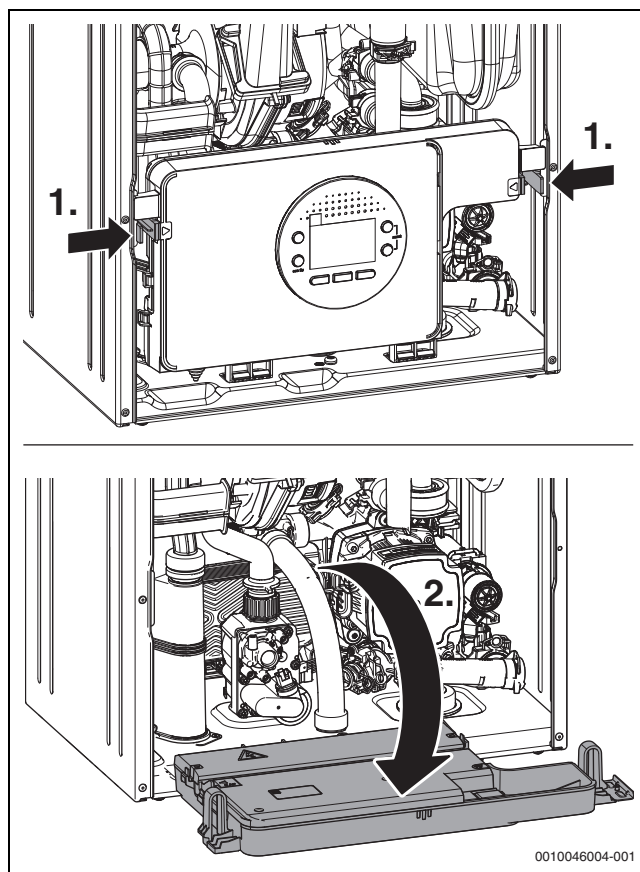
Fig. 31 Rabattre le dispositif électronique
