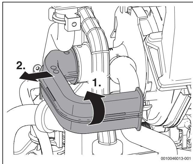
Fig. 111 Démonter le tuyau d'arrivée d'air
