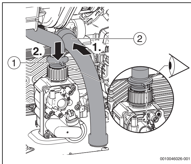
Fig. 147 Monter le tuyau de gaz et le tuyau d'écoulement
