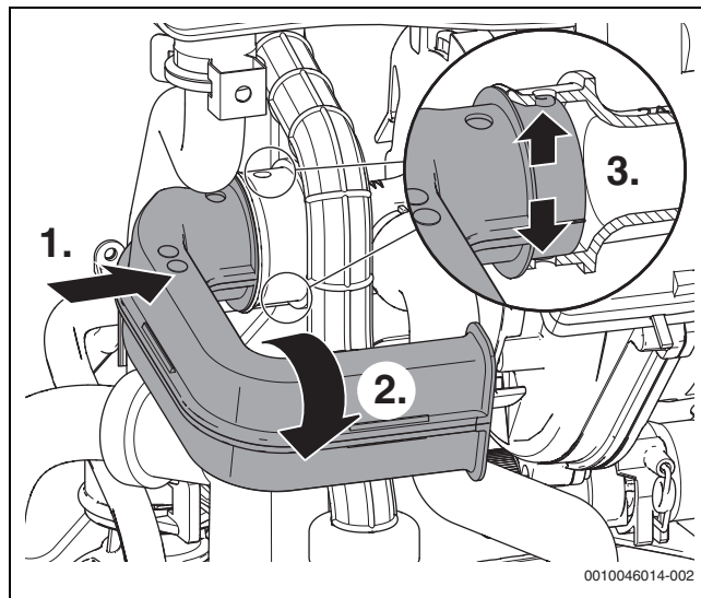
Fig. 112 Monter un nouveau tuyau d'arrivée d'air
