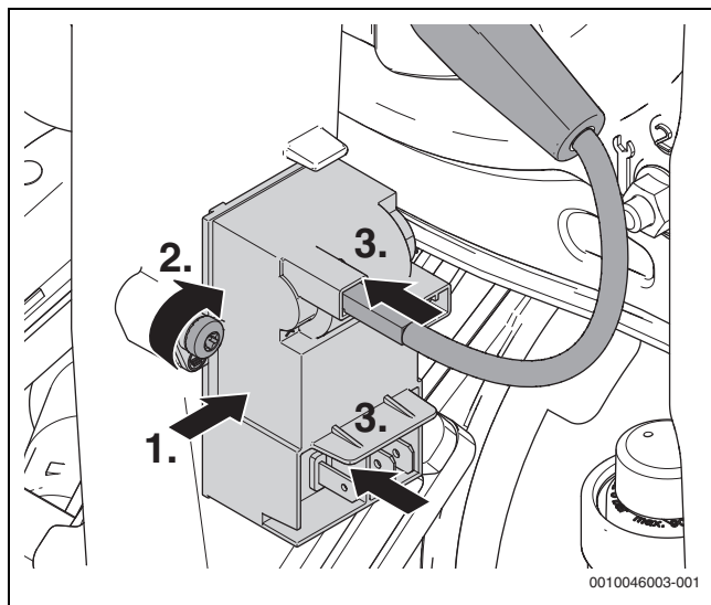
Fig. 110 Monter le nouveau transformateur d'allumage
