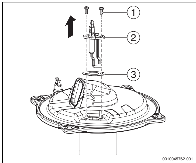
Fig. 70 Démontage de l'électrode d'allumage
