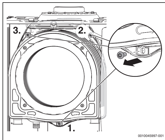
Fig. 105 Démonter l'échangeur thermique
