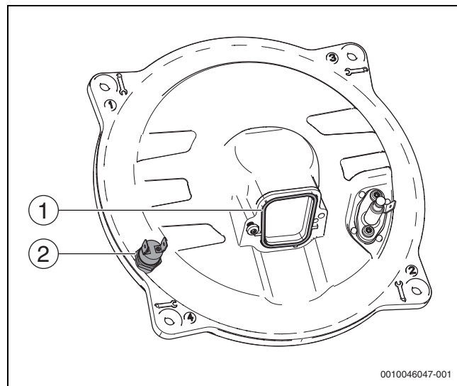
Fig. 128 Composants du module de la porte du foyer
