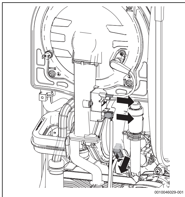
Fig. 116 Débrancher les câbles
