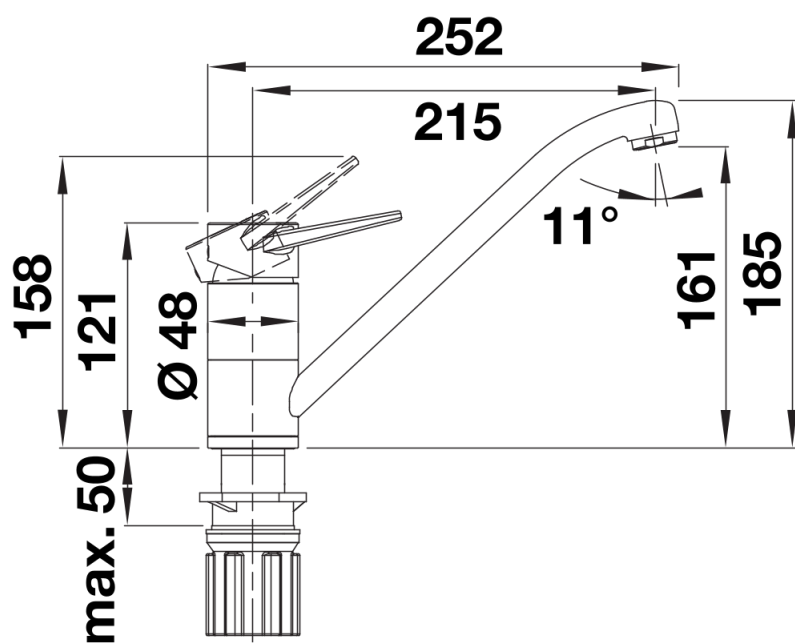
Vue latérale
