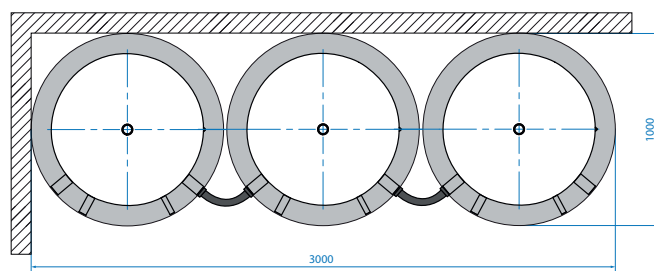
Connexion parallèle
