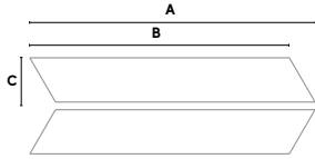
A 11,5 cm - 4 1 / 2 " B 73,6 cm - 29" C 67 cm - 26 3 / 8 "
