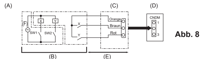
(A) Beispiel eines Schaltplans (B) Anordnung vor Ort X, Y: Relais
