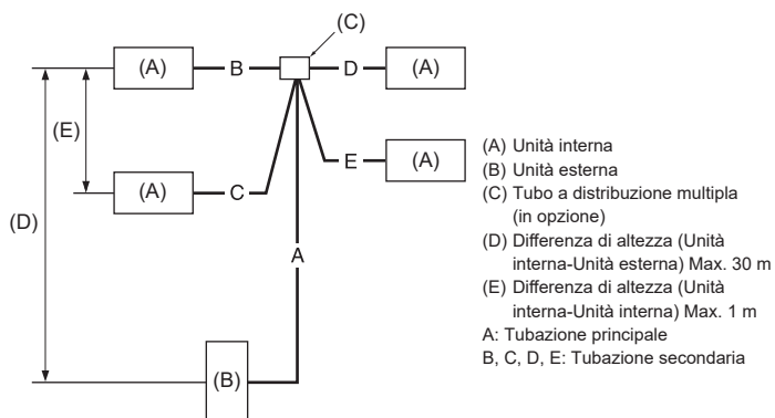
<Limiti dell'installazione della tubazione del refrigerante>
