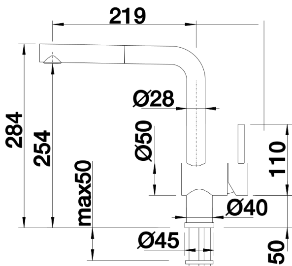
Vue latérale
