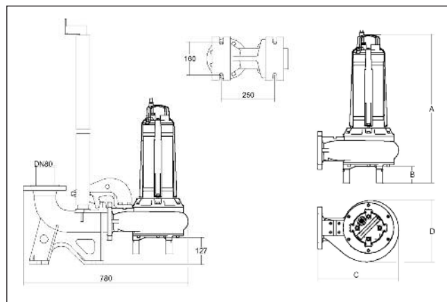
Encombresments (mm)
