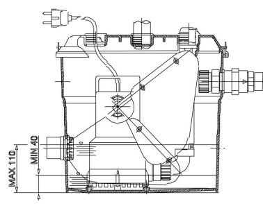
Montage avec flotteur spécial pour bacs à douche
