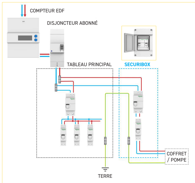
Raccordement électrique monophasé 230V
