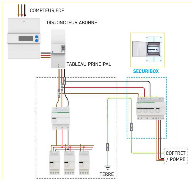
Raccordement électrique triphasé 400V
