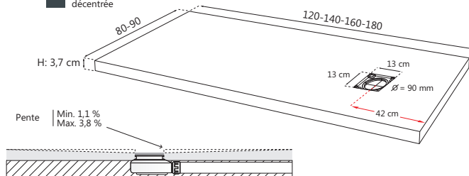
Grille de vidage décentrée
