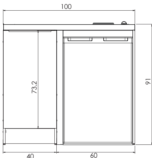
Vue face
