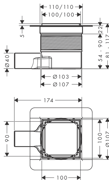
Plan géométral
