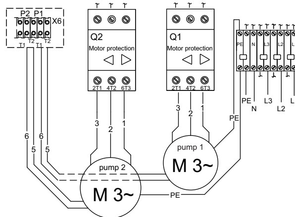
Fig. 14 Multilift MDG
