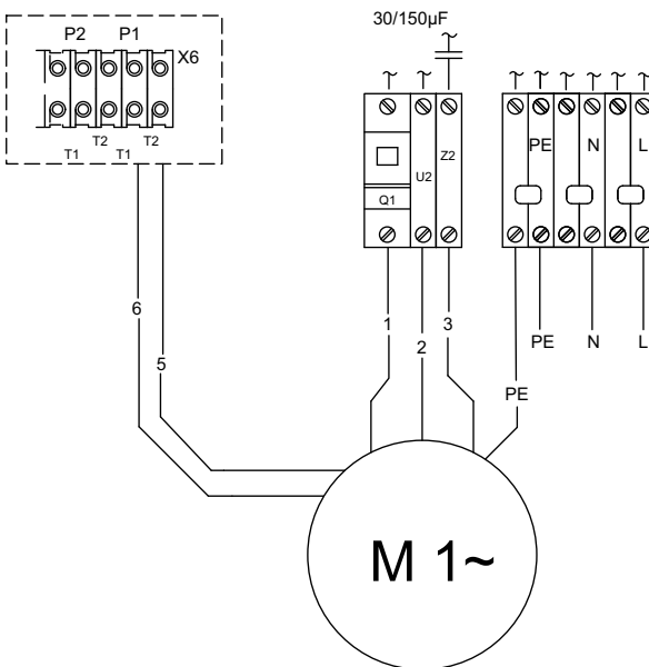
Fig. 11 Multilift MOG
