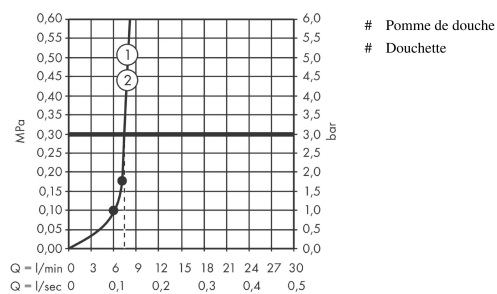
Schéma d'écoulement
