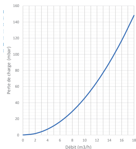
Pertes de charge à débit maximal : 140 mbar
