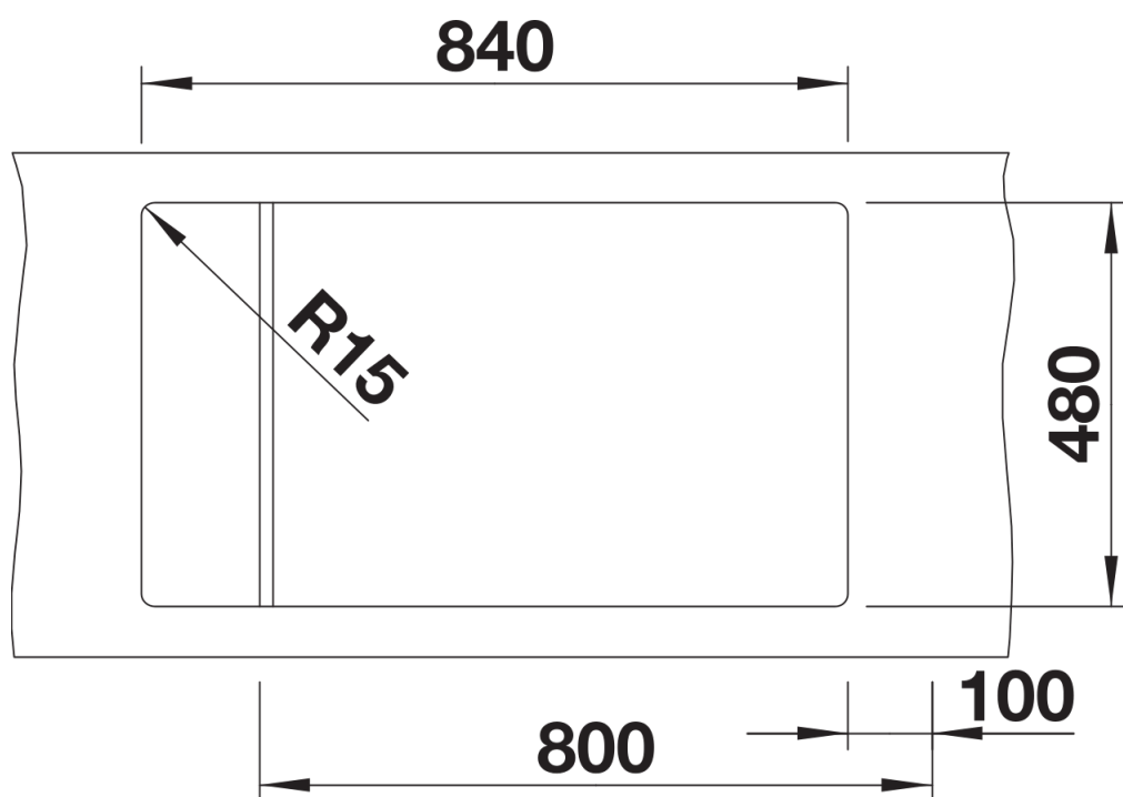
Découpe
