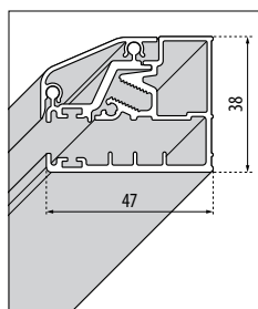
PROFILÉ DE SÉRIE pour panneau fixe
