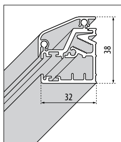
PROFILÉ DE SÉRIE pour GALA A / G / 1B / 2P
