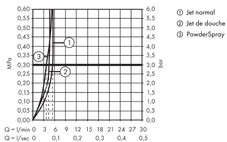
Schéma d'écoulement
