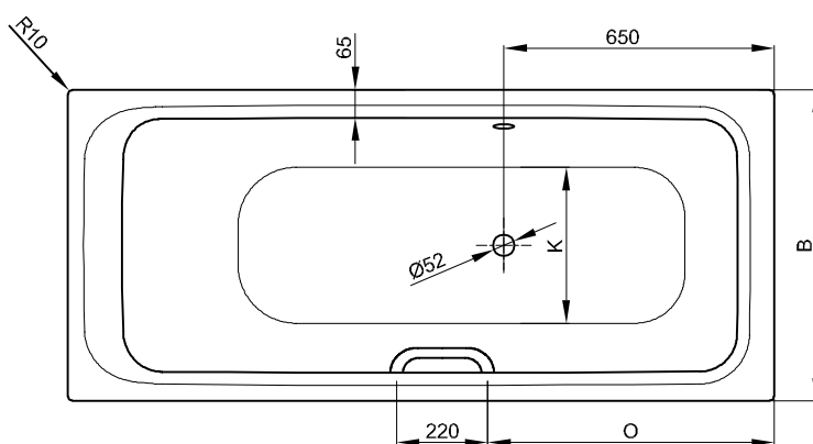
N° 2: trop-plein latéral à gauche
