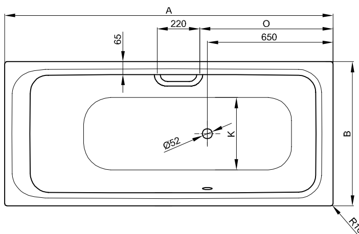
N° 1: trop-plein latéral à droite
