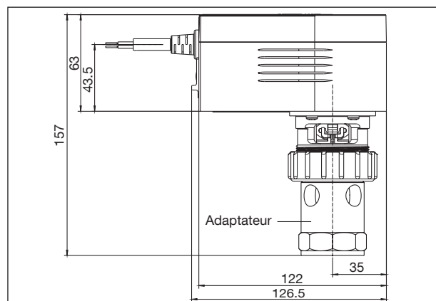
Encadrements avec adaptateur monté
