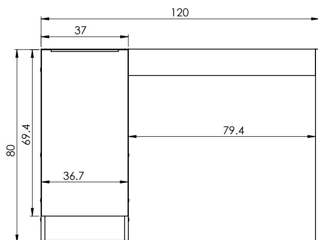
Vue face
