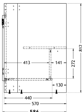
VUE DE DROITE (Semelle réduite)
