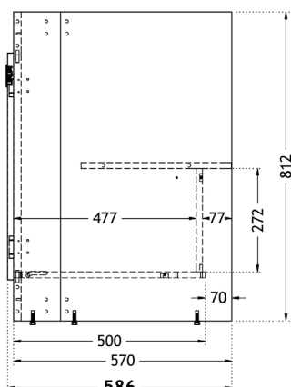
VUE DE DROITE (Poubelle sélective)
