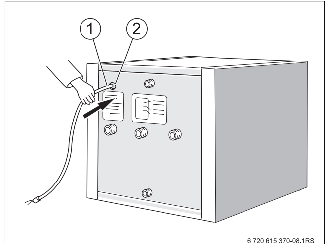
Afb. 9 Monteer de warmwatertemperatuursensor
