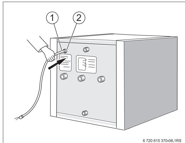
Bild 9 Warmwasser-Temperaturfühler montieren
