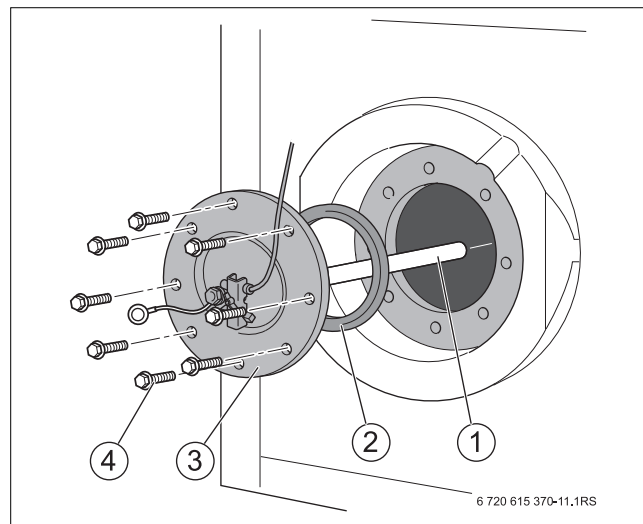
Sl. 13 Otvaranje otvora za ispitivanje
