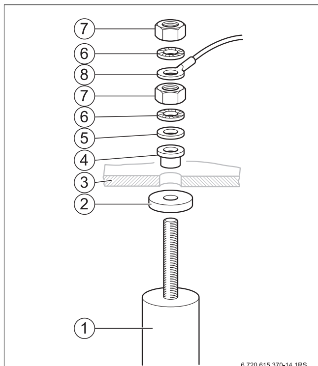
Bild 15 Magnesium-Anode prüfen
