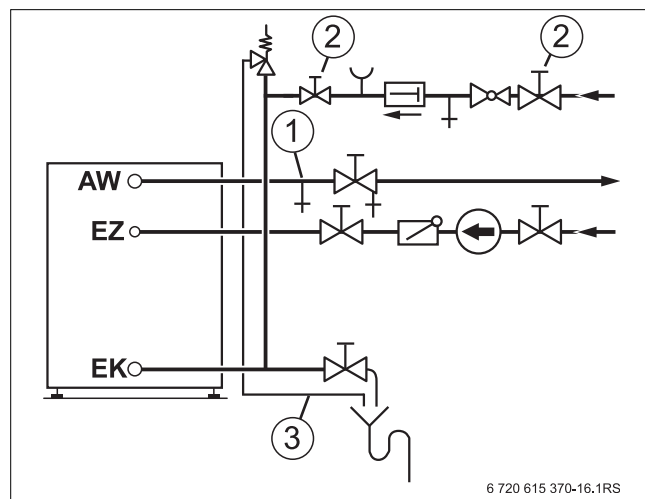
Sl. 11 Ispitivanje nepropusnosti
