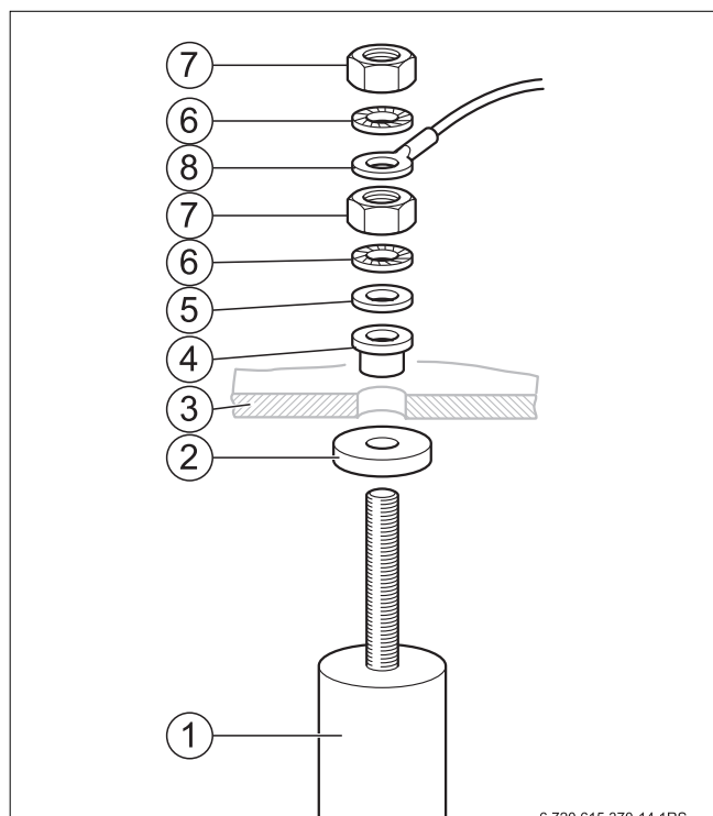
Fig. 15 Comprobación del ánodo de magnesio
