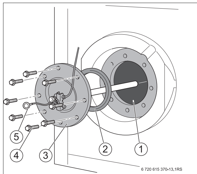
Bild 16 Prüföffnung schließen
