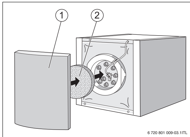
Fig. 12 Montaje del aislamiento térmico y la pared delantera
