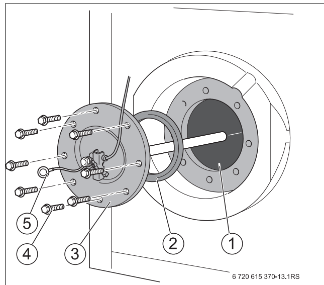
Fig. 16 Fermer la trappe de visite
