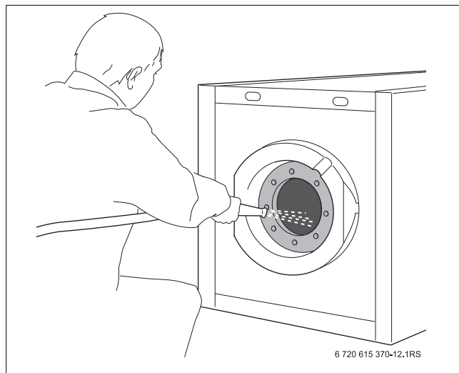
Afb. 14 Warmwaterboiler uitspuiten
