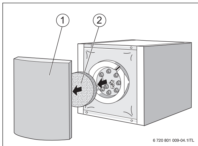
Bild 8 Vorderwand und Wärmeschutz abnehmen
