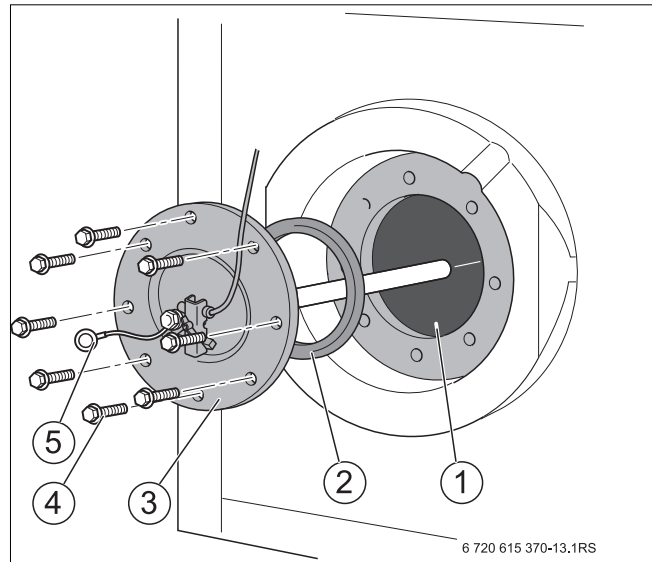
Afb. 16 Inspectieopening sluiten
