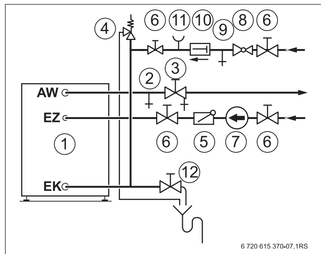
Afb. 7 Installatie (principeafbeelding)
