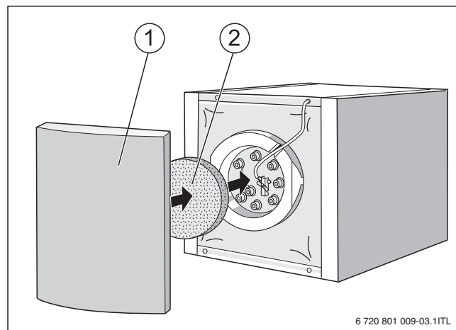
Afb. 12 Monteer isolatie en voorwand
