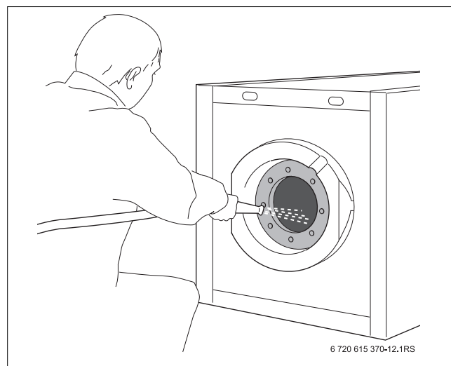
Sl. 14 Prskanje spremnika tople vode
