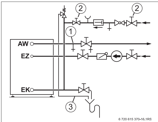
Bild 11 Dichtheit prüfen
