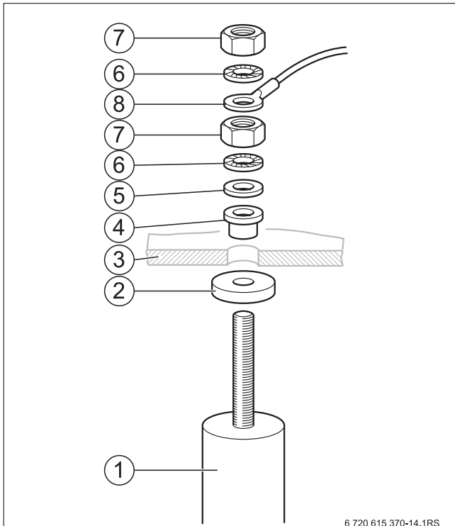
Afb. 15 Magnesiumanode controleren
