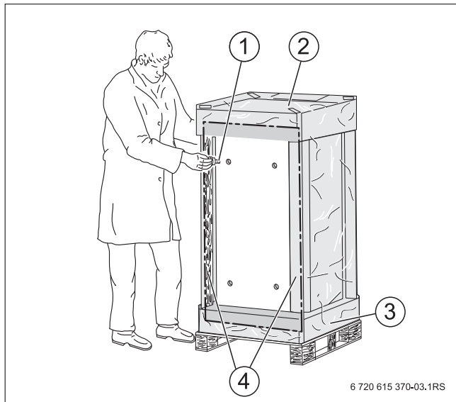
Afb. 3 Snijd de verpakkingsfolie open en breng de voetschroeven aan
