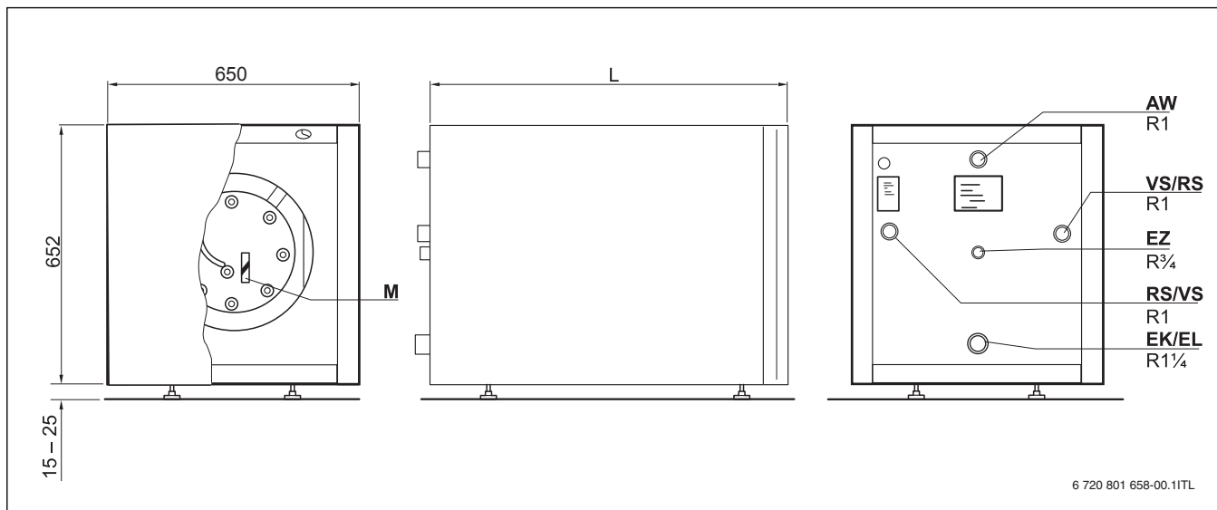
Sl.2 Izvedbene i priključne dimenzije WST 135-2 HRC, WST 160-2 HRC i WST 200-2 HRC
