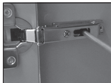
Réglage en hauteur Height adjustment Höheneinstellung
