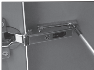
Réglage en profondeur Depth adjustment Tiefeneinstellung
