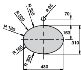
Plan de découpe Encastrement par dessus
