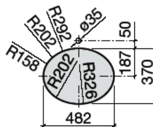
Plan de découpe Encastrement par dessus
