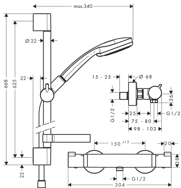
Plan géométral
