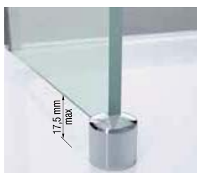
PIED DE FIXATION SUR RECEVEUR Ø 29 MM
