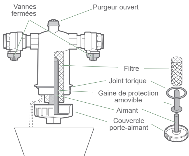
fig. 17 - Nettoyage du pot à boues
