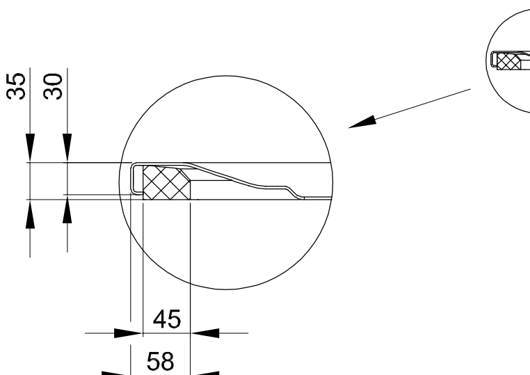
Présentation avec Support Minimum prémonté (T1).
