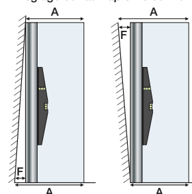
Réglage du faux-aplomb du mur
