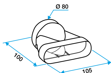
Raccord mixte pour conduit Ø80 mm
