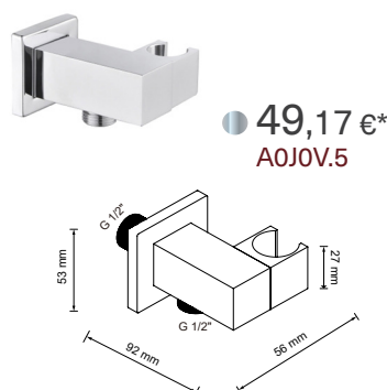
COUDE DE SORTIE EN LAITON
